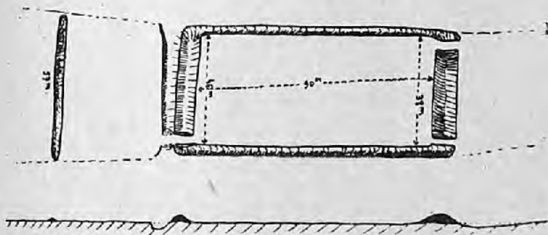
Fig. 2. - Plan et coupe du Pouyoulet
